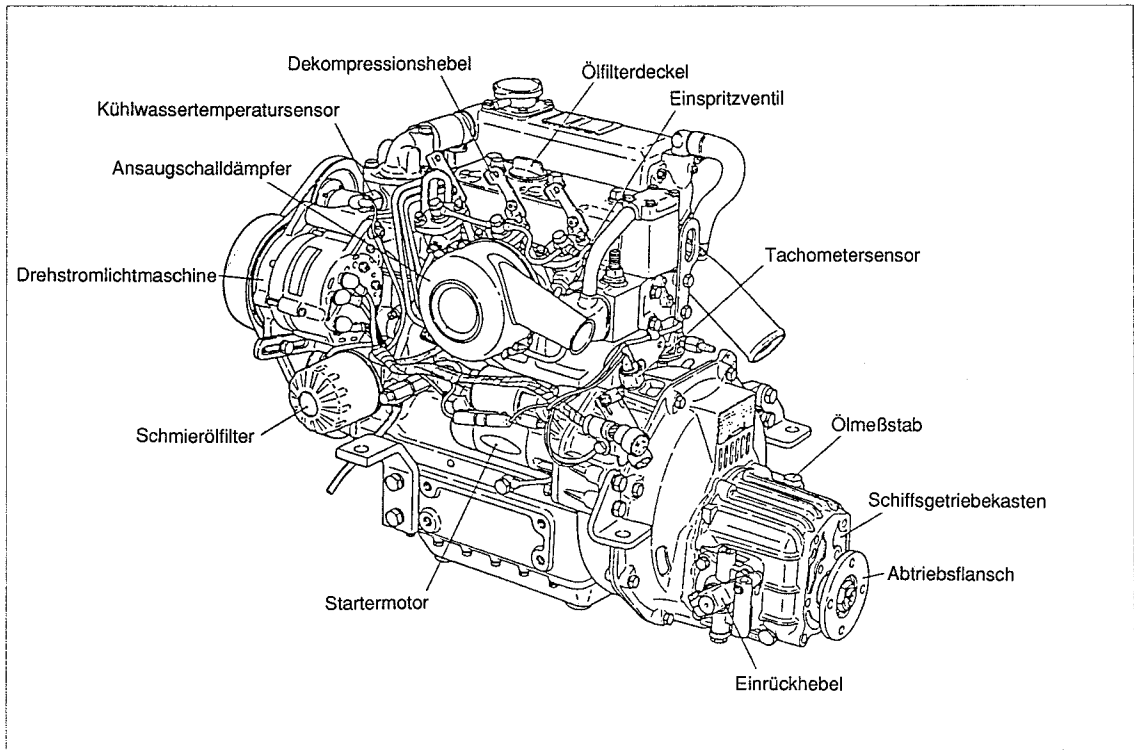
Ansaugseite 3GM30F
