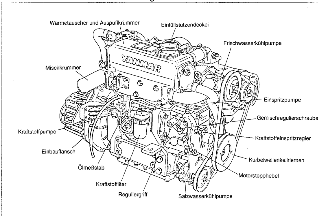
Auspuffseite 3GM30F
